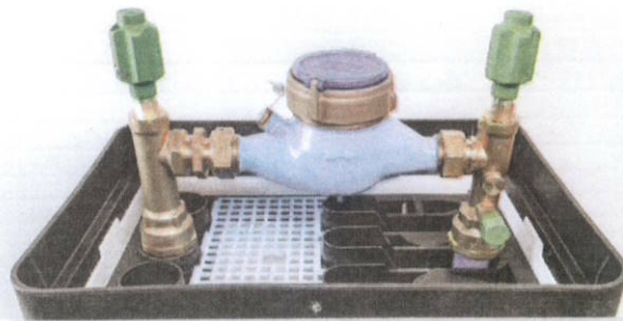
MODULO 1 V: Ventil před i za vodoměrem, včetně zpětné klapky s odvzdušněním, pro vodoměr DN20 (závit 1")
